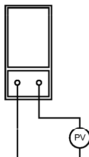
Рисунок 1 — Схема измерения напряжения холостого хода
